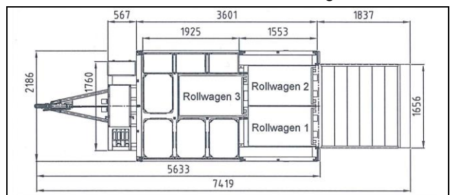
Ausführung mit 3 Rollwagen
