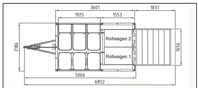
Ausführung wahlweise mit 2 Rollwagen
