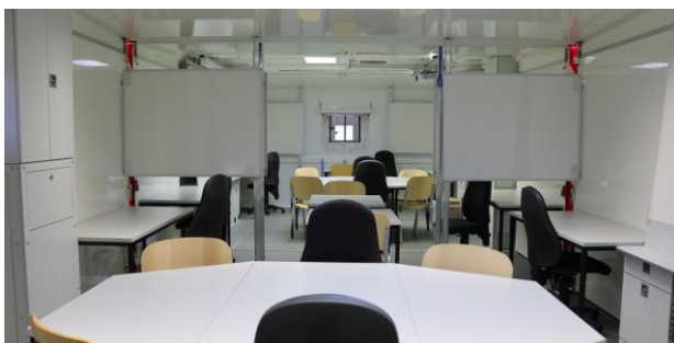
Blick Innenraum: zwei miteinander verbundene AnhFüLa
